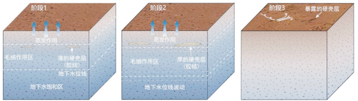
祝融号在着陆区发现富含含水矿物的板状硬壳层及其在地下水作用下的形成过程示意图。(国家航天局提供)
